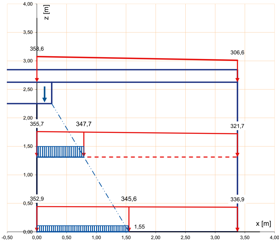
Belastungsbild
