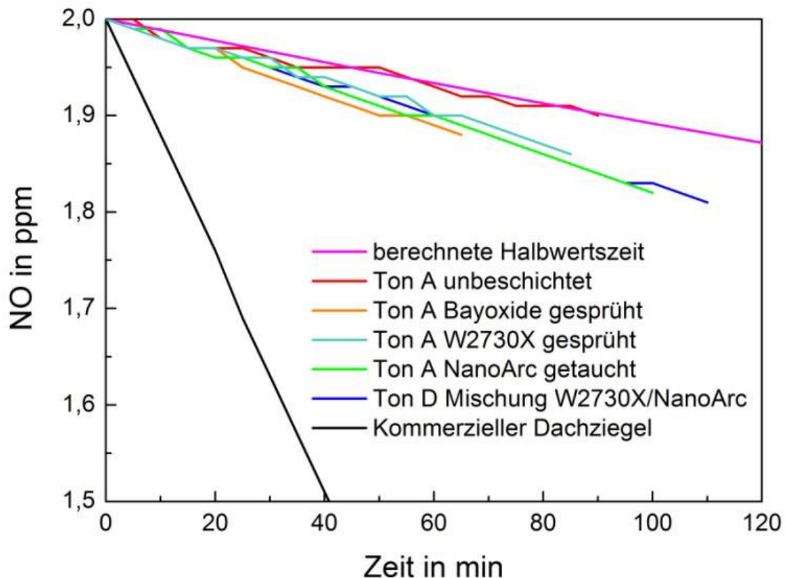
Abb. 1: NO-Abbau verschiedener Beschichtungen verglichen mit dem Referenzziegel
